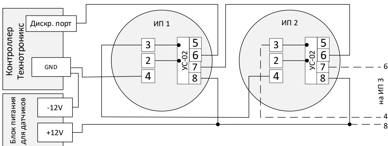
Рис.5.2. Схема подключения ИП212-141 с УС-02 к дискретному входу контроллера
