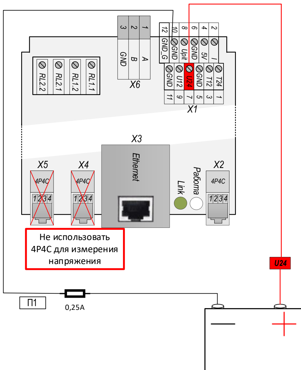
Рис.4.4. Схема подключения одной АБ 12В к разъему X1 (измерение напряжения)
