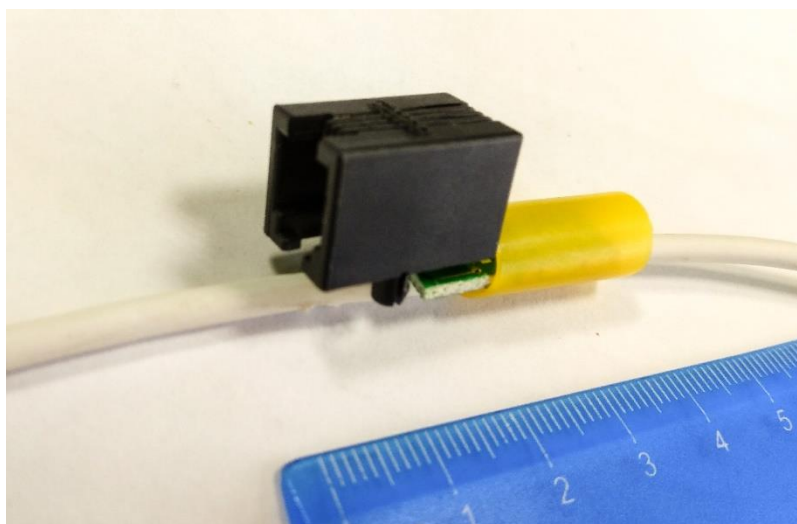
Рис.7.1. Внешний вид датчика тока Л20
