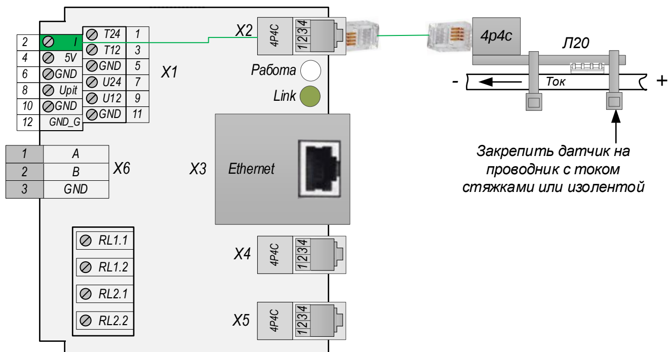
Рис.7.2. Монтаж и схема подключения датчика тока Л20. Вариант 1
