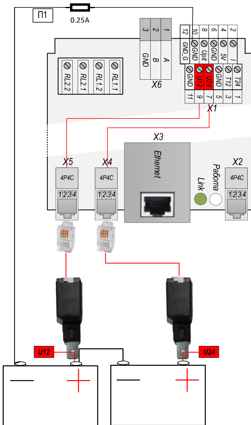
Рис.4.1. Схема подключения двух АБ 12В к разъемам X5, X4 (измерение напряжения и температуры)
