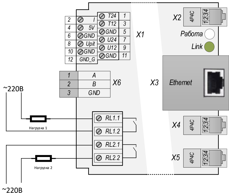
Рис.6.1. Подключение нагрузки на оптореле RLX.X.
