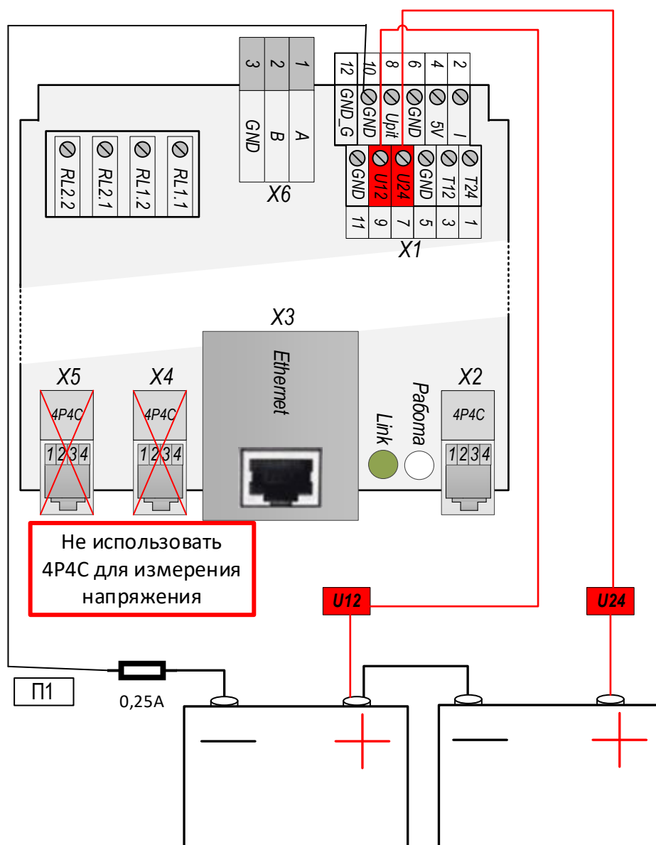
Рис.4.3. Схема подключения двух АБ 12В к разъему X1 (измерение напряжения)
