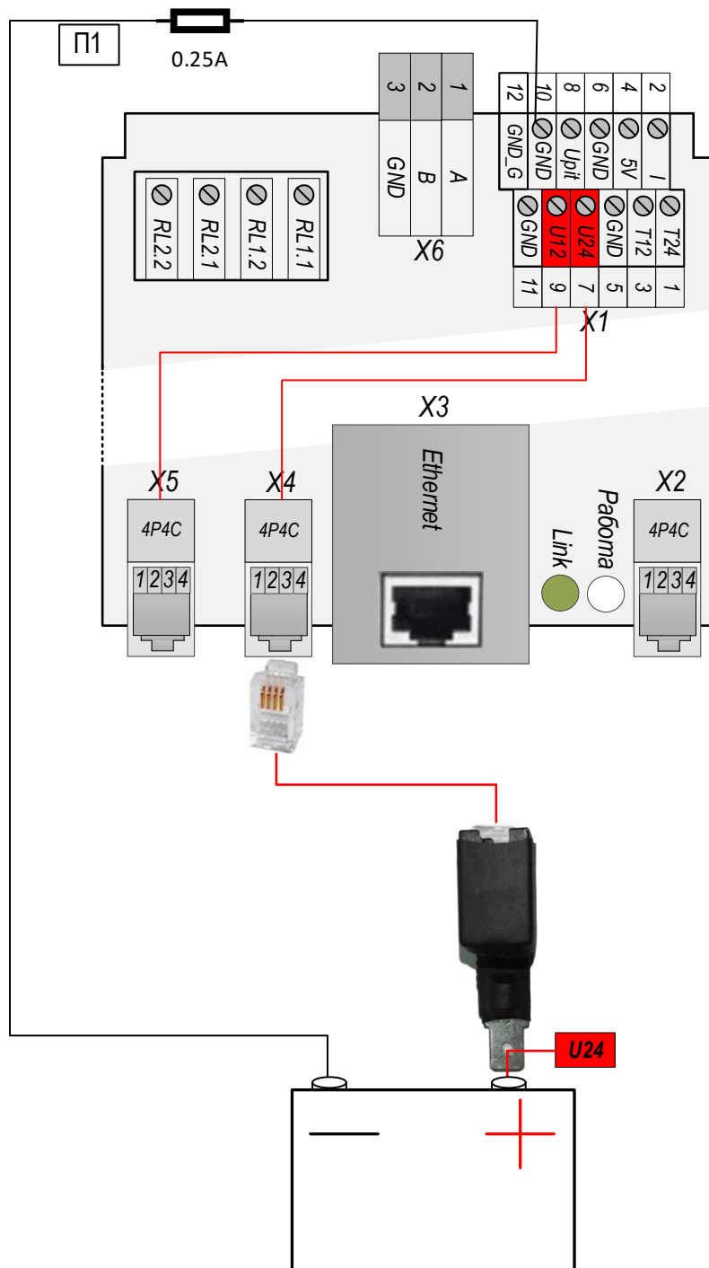
Рис.4.2. Схема подключения одной АБ 12В к разъему X4 (измерение напряжения и температуры)
