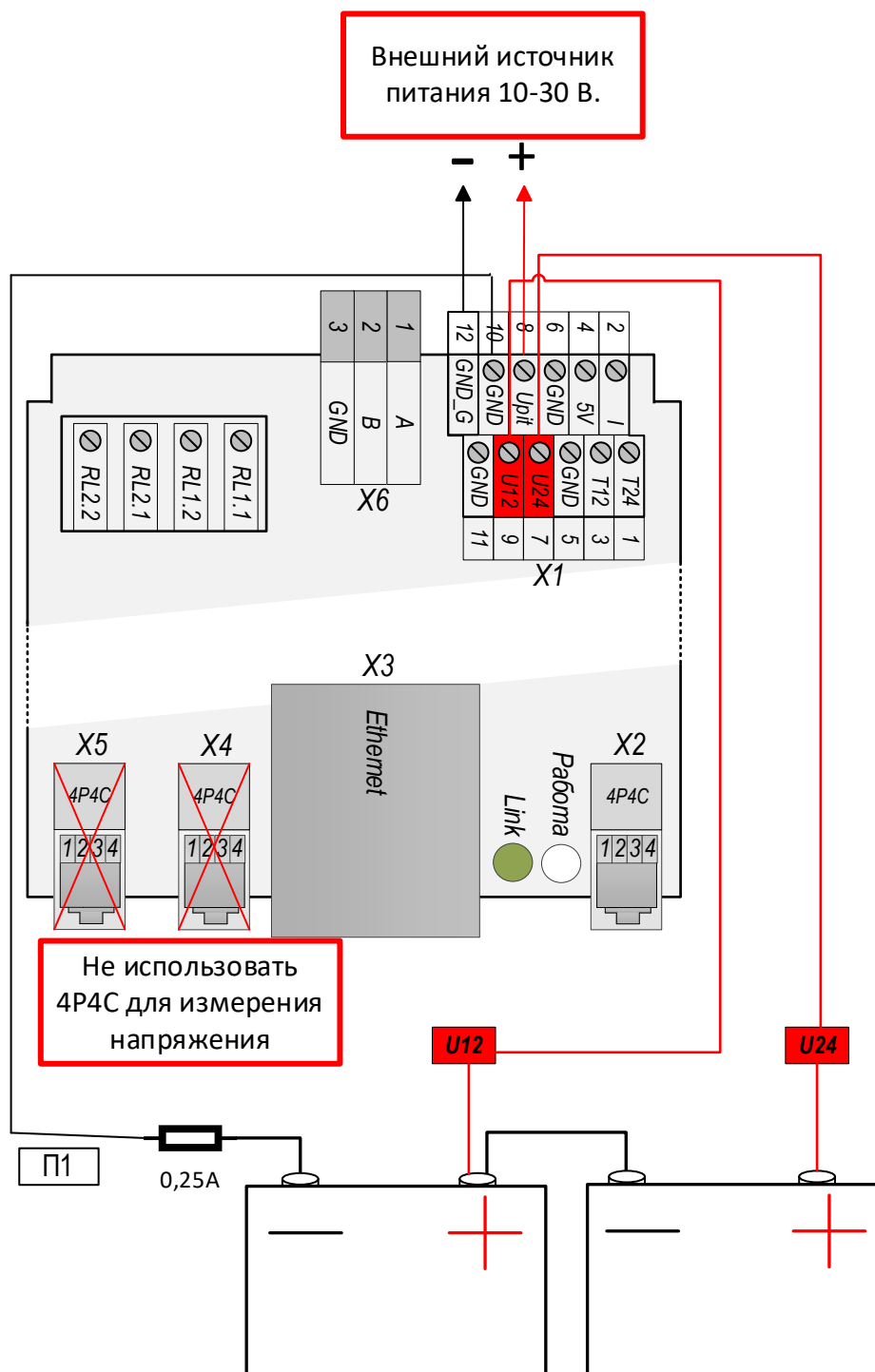
Рис.2.1. Пример подключения питания от внешнего источника с гальванической развязкой
