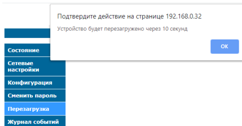
Рис.10.7. Страница «Перезагрузка».
