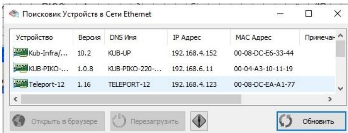
Рис.9.1. Утилита «picSearch»
