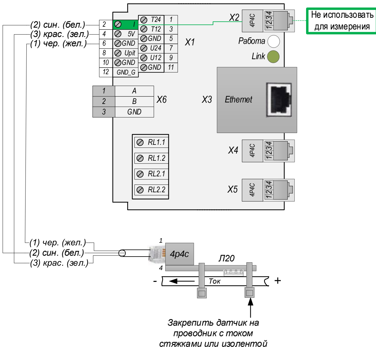
Рис.7.3. Монтаж и схема подключения датчика тока Л20. Вариант 2
