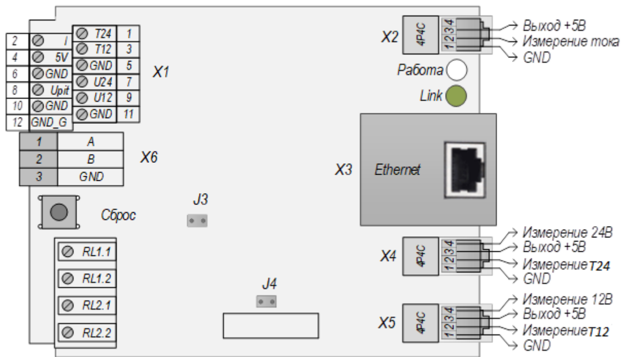
Рис.1.1. Функциональные элементы изделия
