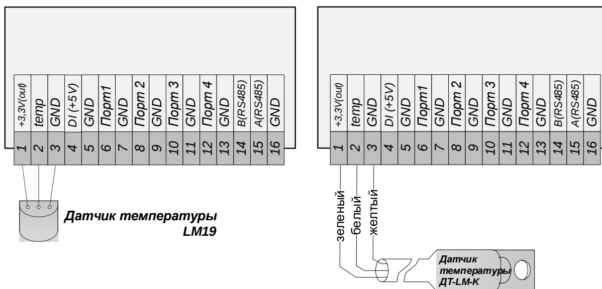
Рис.4.1. Подключение датчиков температуры LM19 (слева) и ДТ-ЛМ-К (справа)
