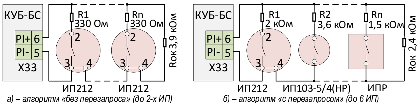
Рис. 32 Подключение активных и пассивных ИП с Нормально Разомкнутыми контактами по двухпроводной схеме. (Номера контактов извещателей указаны для ИП212-141, 41М, 45 и т.н.)
