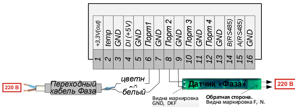
Рис.6.1. Подключение «Переходного кабеля Фаза» (слева) или «Датчика фазы» (справа), Пример для портов №1 и №2
