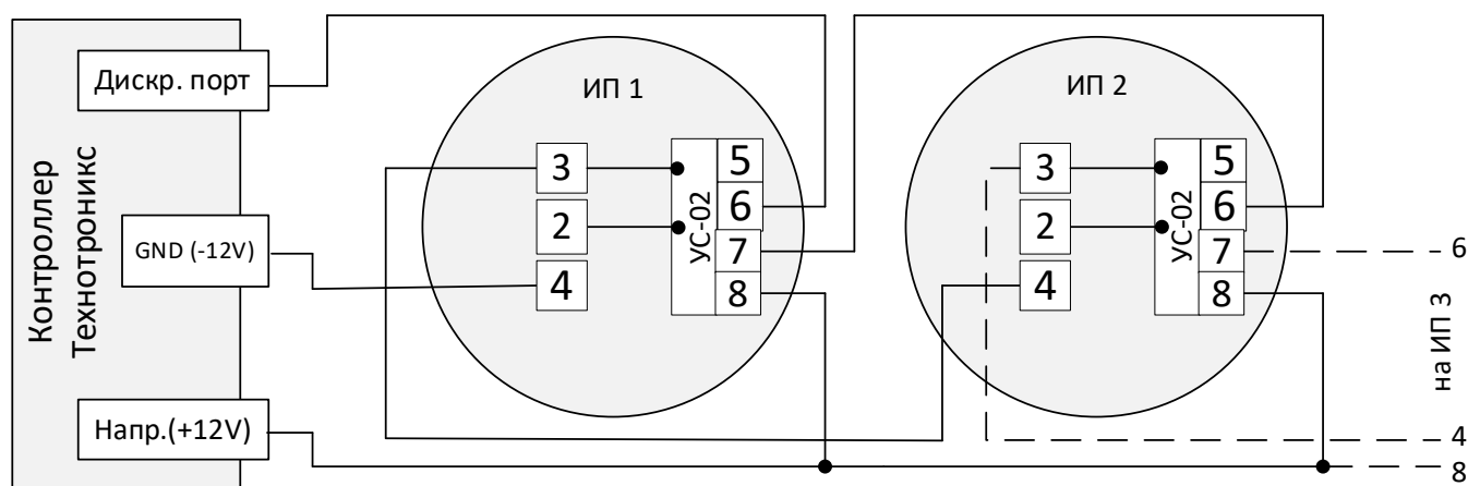
Рис.5.2. Схема подключения ИП212-141 с УС-02 к дискретному входу контроллера
