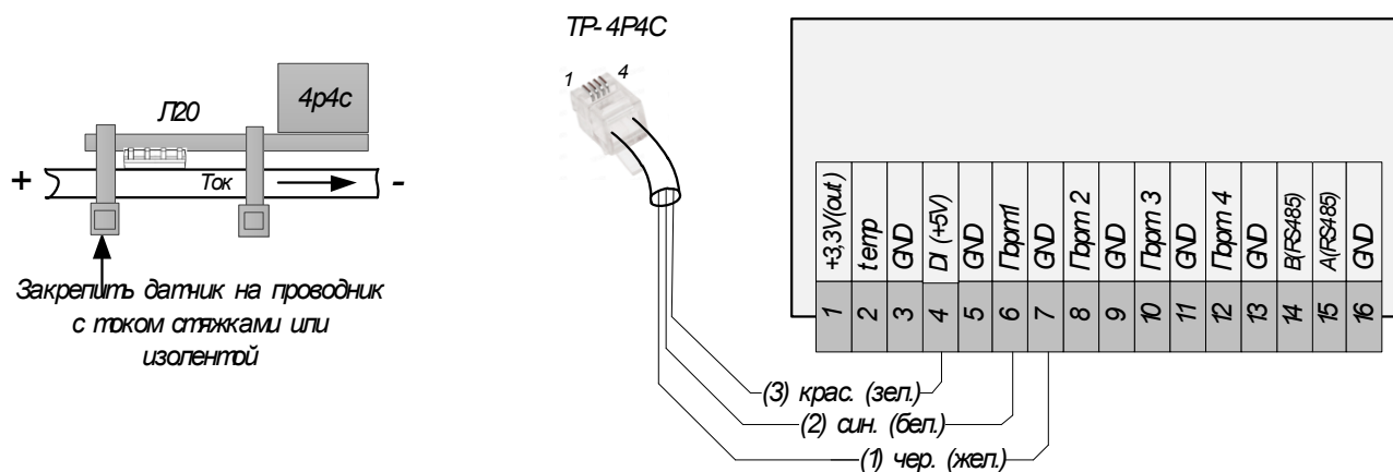
Рис.8.2. Монтаж (слева). Подключение датчика тока Л20 (справа, остальные типы аналогично)
