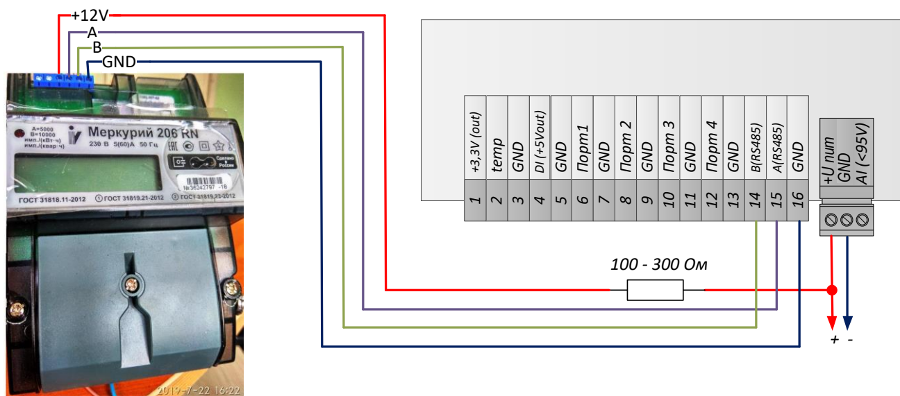
Рис.11.3. Пример подключения к интерфейсу RS-485 электросчетчика «Меркурий 206RN» или PRNO. (У счетчиков «Меркурий 206 PRSN» или PRSNO цепь +12V подключать не требуется).
