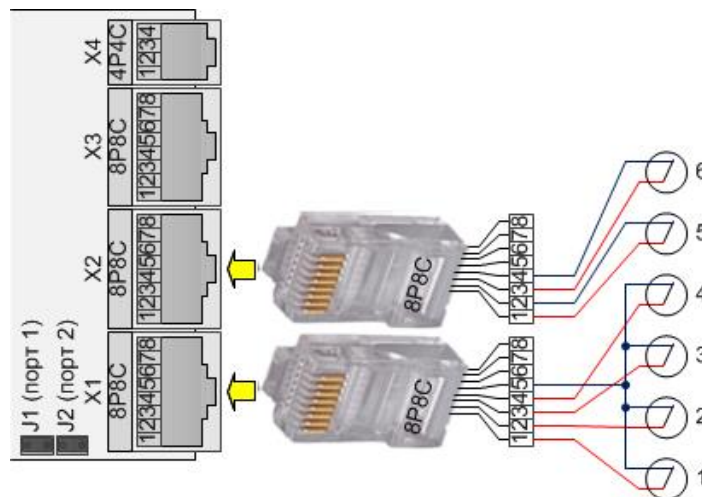
Рис.8. Подключение к входам сухой контакт
