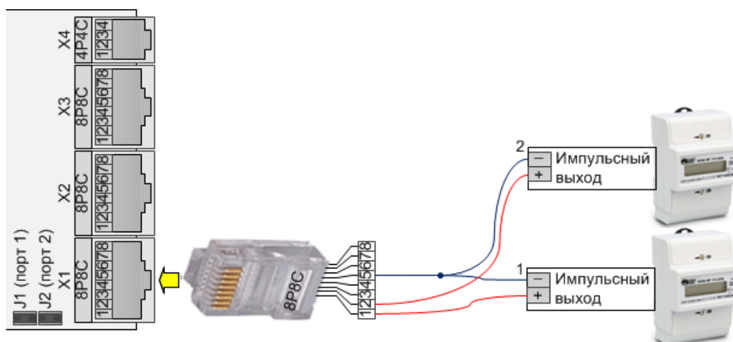
Рис.26. Подключение к входам счетчика импульсов
