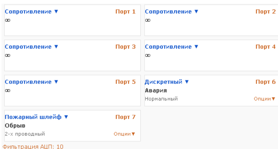
Рис.25. Конфигурация портов в качестве входов измерения сопротивления
