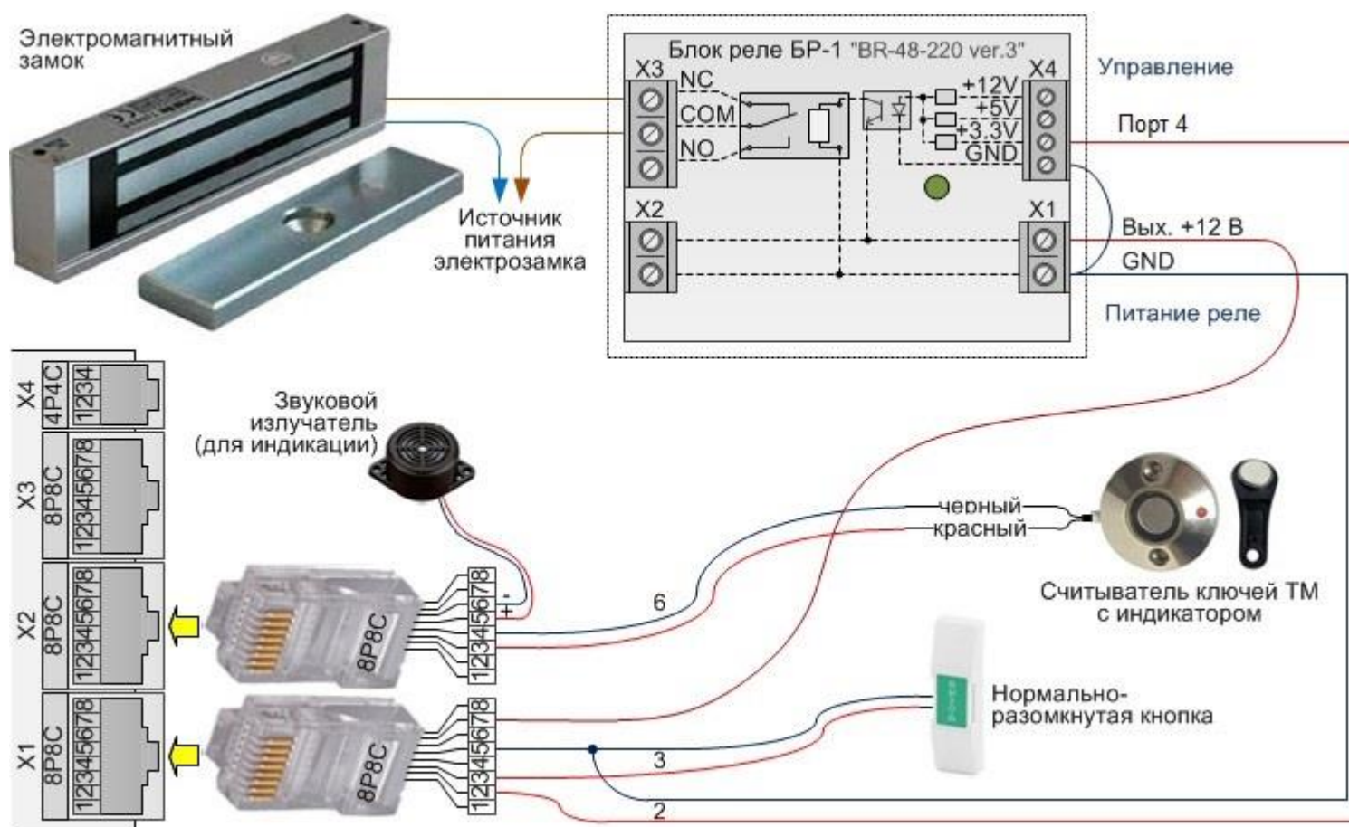
Рис.42. Схема для автоматического управления электрозамком
