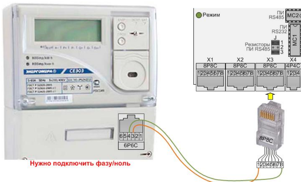
Рис.59. Схема подключения электросчетчика Энергомера CE303 S34 *А*
