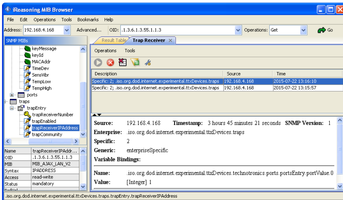
Рис.71. Получение трапа о сработке входа изделия
