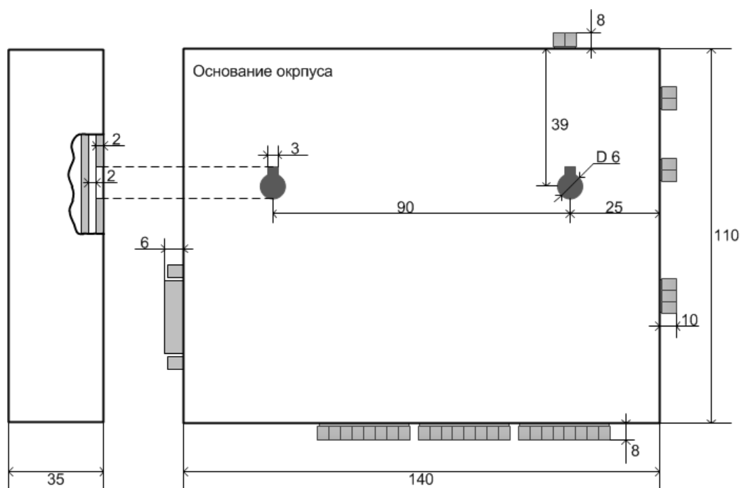
Рис. 26. Основание корпуса изделия с монтажными отверстиями
