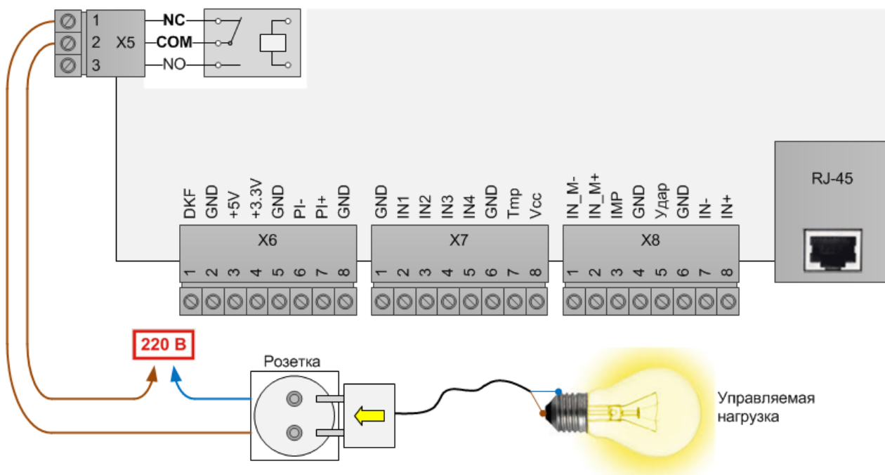
Рис. 13. Реле в нормально-замкнутых цепях питания
