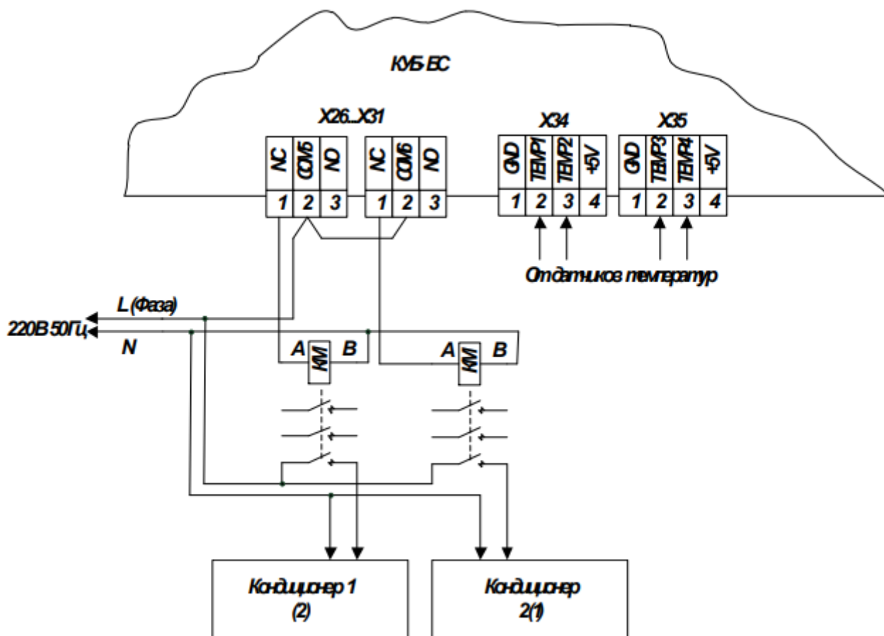
Рис. 33 Подключение кондиционеров к КУБ-БС
