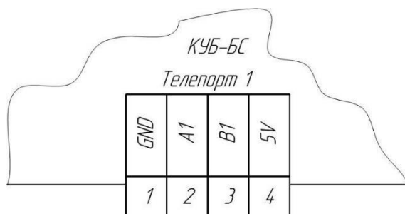
Рис. 15. Назначение контактов клеммников интерфейса RS-485
