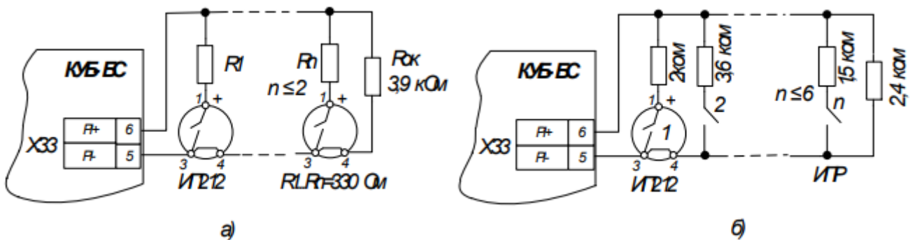
Рис. 30 Подключение активных и пассивных ПИ с НО-контактом по двухпроводной схеме а) – алгоритм «без перезапроса», б) – «с перезапросом»
