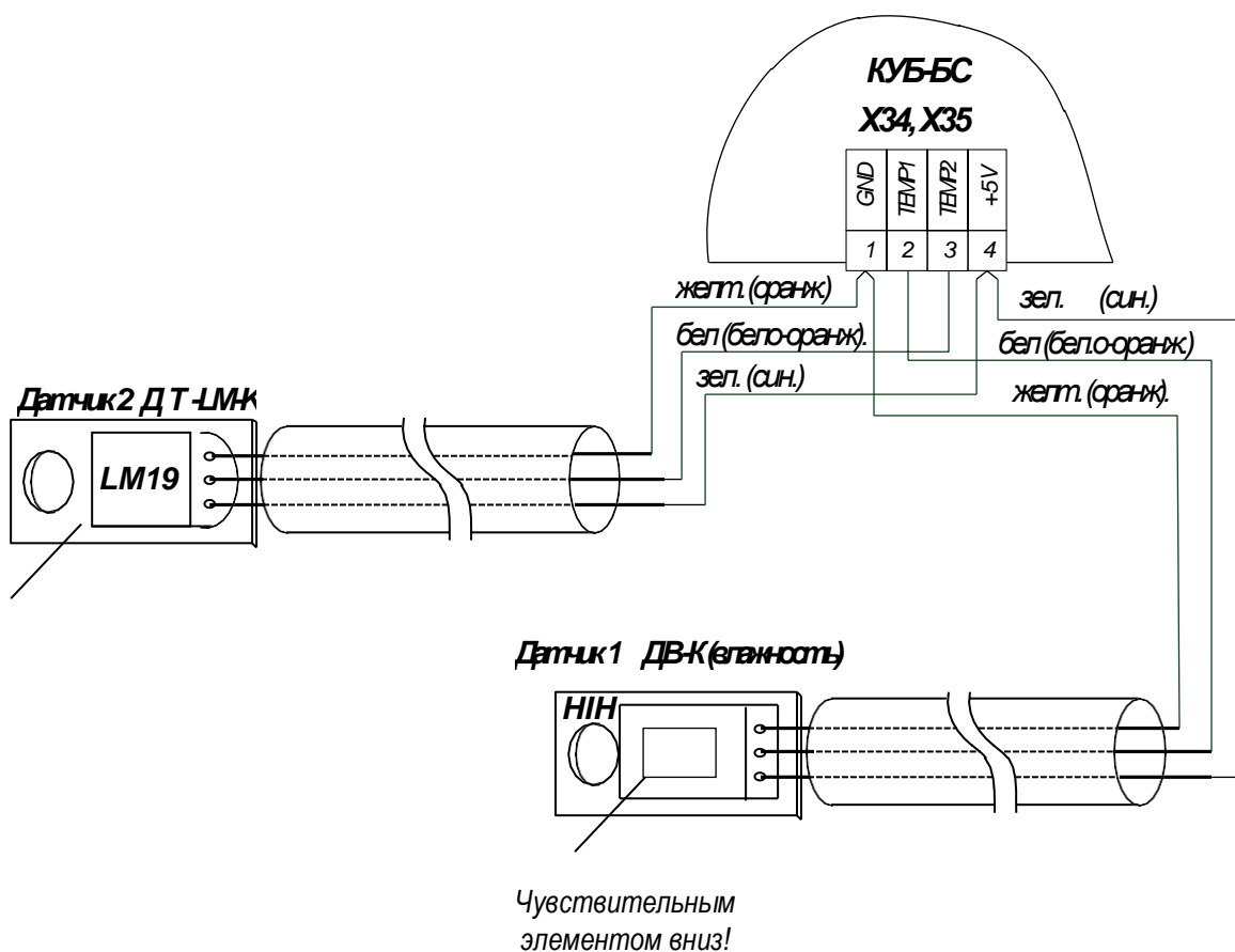
Рис. 32 Пример подключения датчиков температуры и влажности к КУБ-БС
