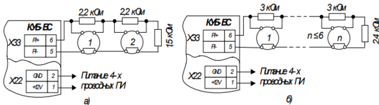
Рис. 31 Подключение активных и пассивных ПИ с НЗ-контактом по четырехпроводной схеме а) – алгоритм «без перезапроса», б) – «с перезапросом»
