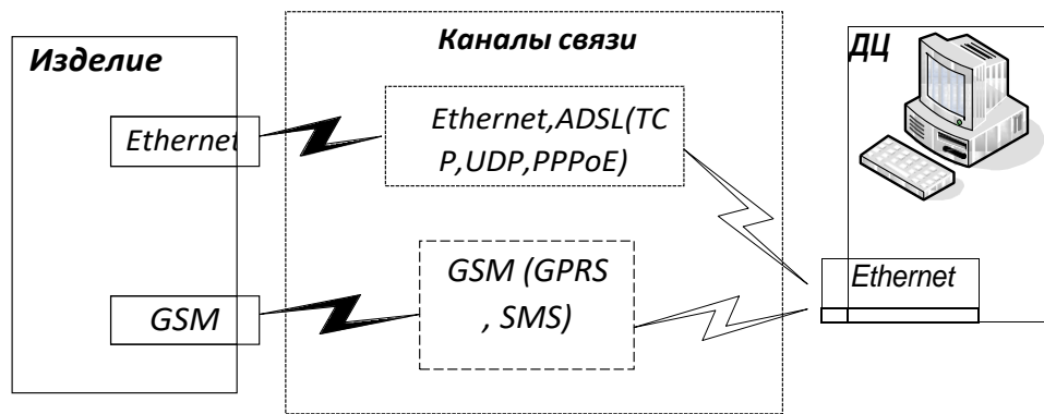
Рис.3. Каналы связи изделия с ДЦ*
