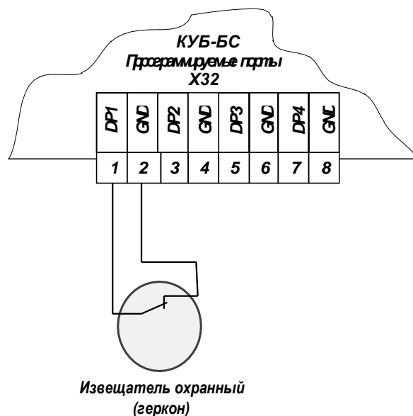
Рис. 26 Подключение датчика к программируемому порту
