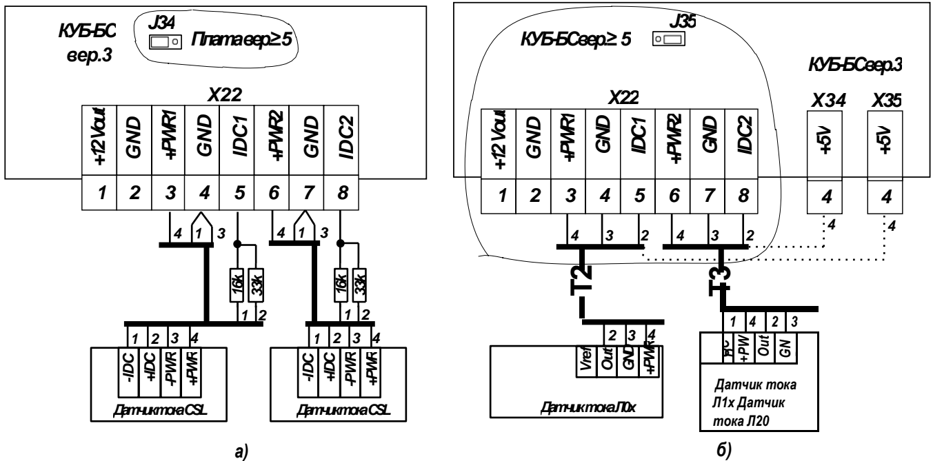
Рис. 20 Подключение к контроллеру датчиков тока CSL (а), Lxx (б)
