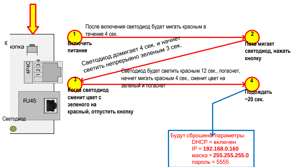
Рисунок 12. Алгоритм применения кнопки сброса
