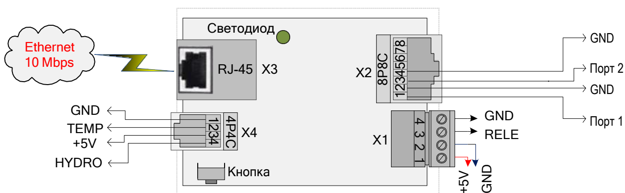
Рисунок 1 а. Схема размещения функциональных элементов на плате ver. 2
