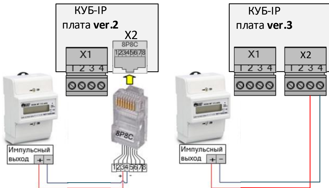
Рисунок 7. Подключение импульсному выходу прибора учета.
