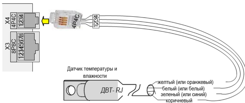
Рисунок 3. Подключение датчика «Кабель ДВТ-RJ»
