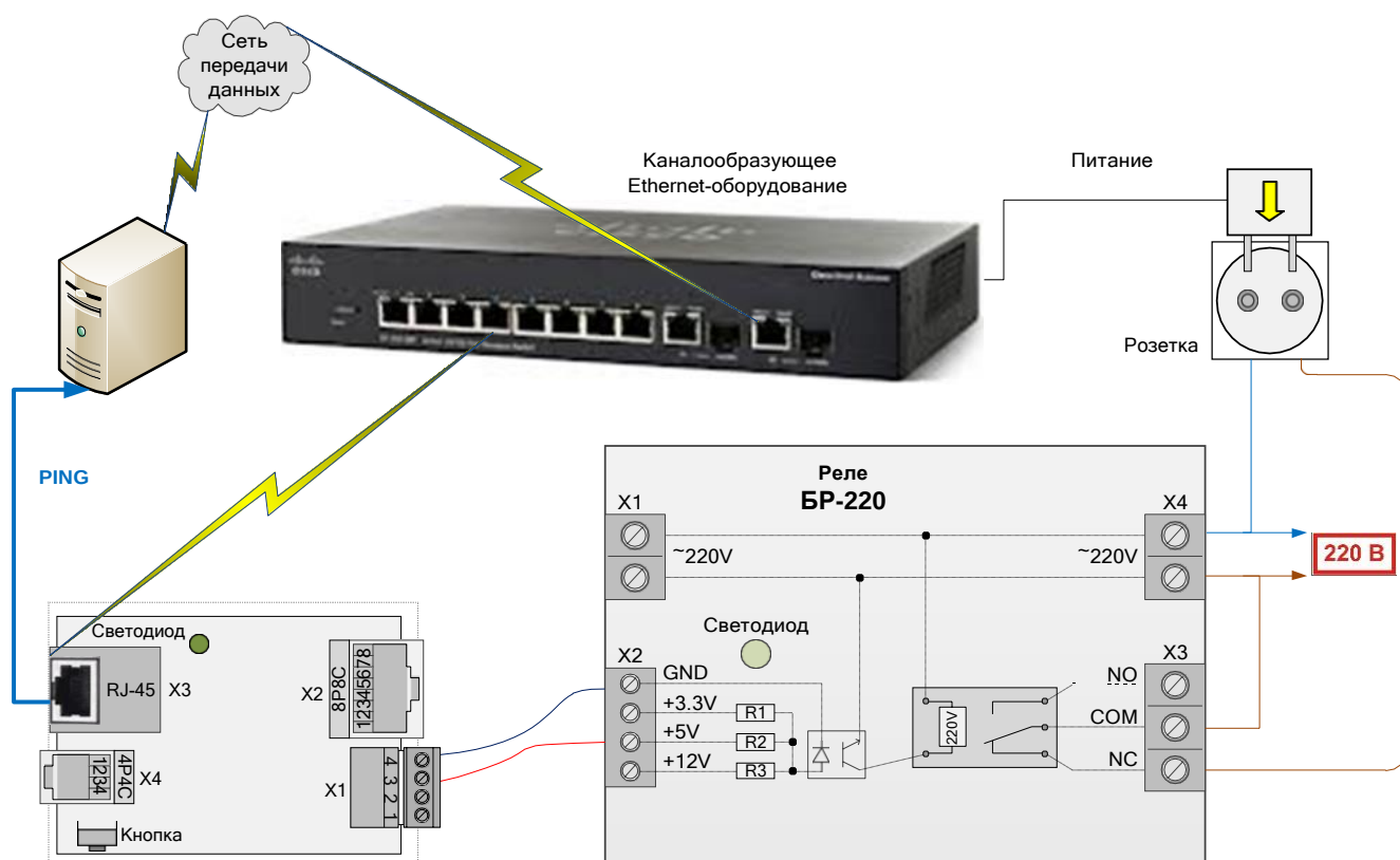
Рисунок 11. Схема перезапуска зависающего сетевого оборудования
