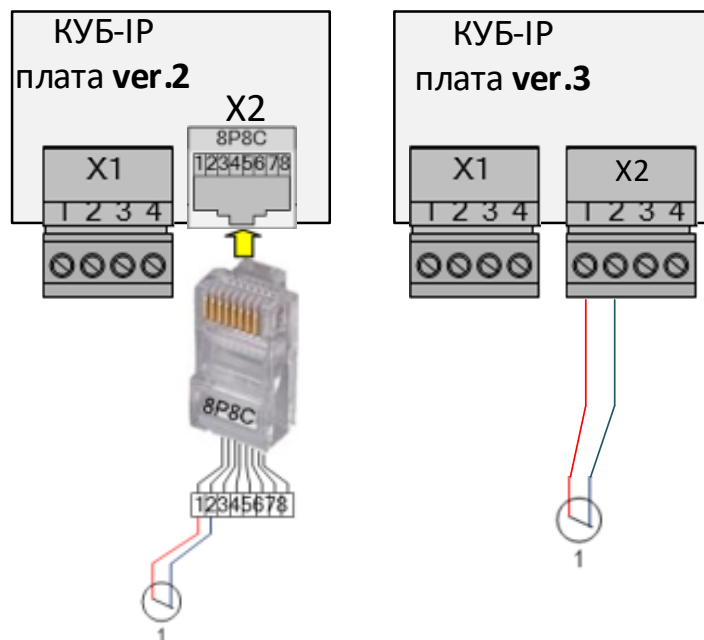
Рисунок 4. Подключение датчиков с выходом сухой контакт
