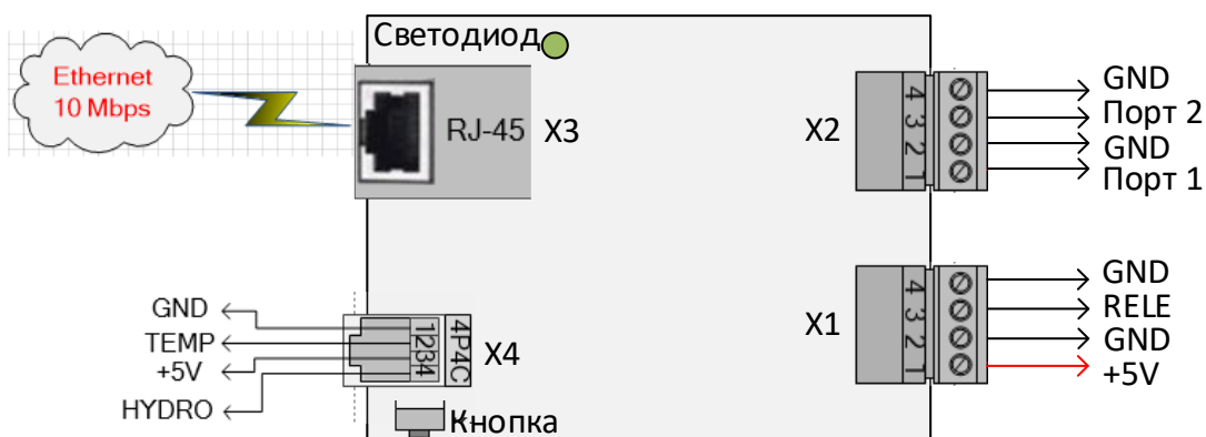
Рисунок 1 б. Схема размещения функциональных элементов на плате начиная с ver. 3
