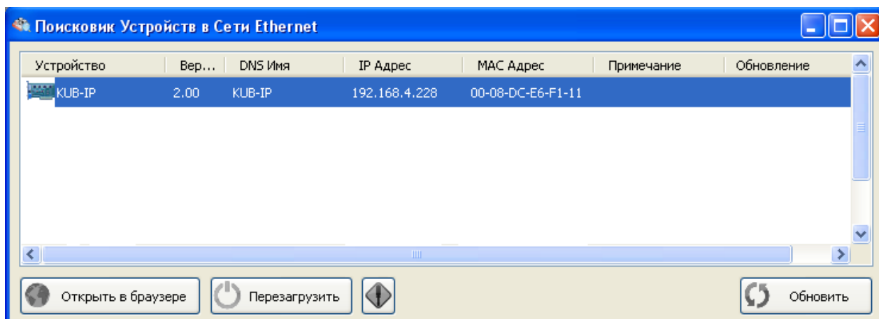
Рисунок 13. Утилита pic-search.exe
