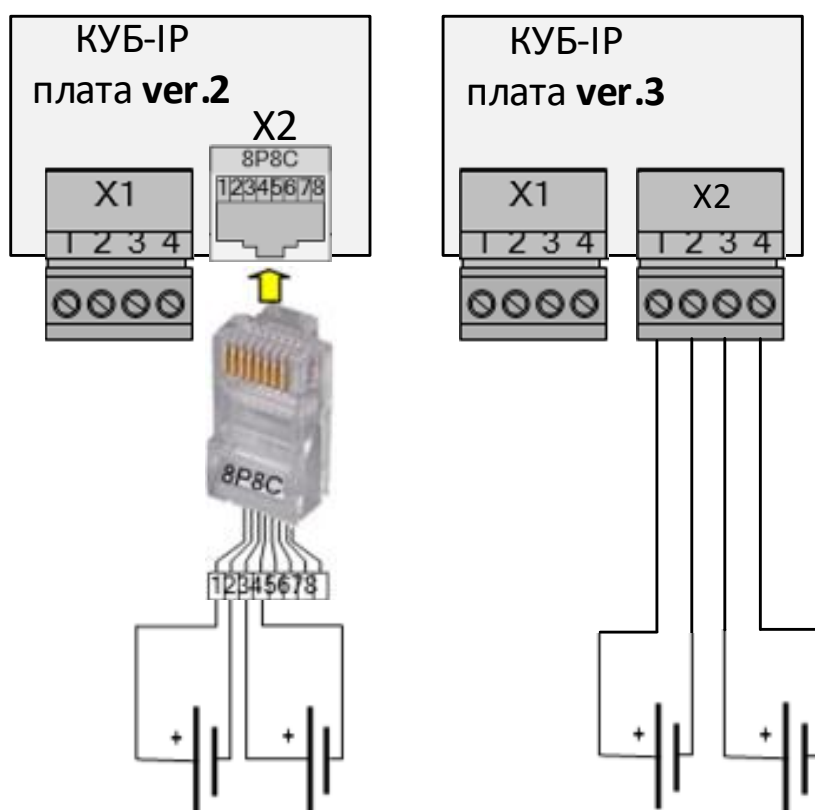
Рисунок 8. Подключение портов для измерения уровня напряжения
