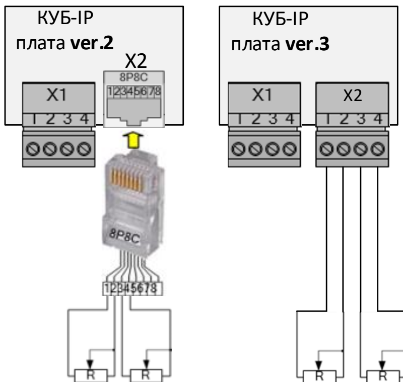
Рисунок 9. Подключение портов для измерения уровня сопротивления
