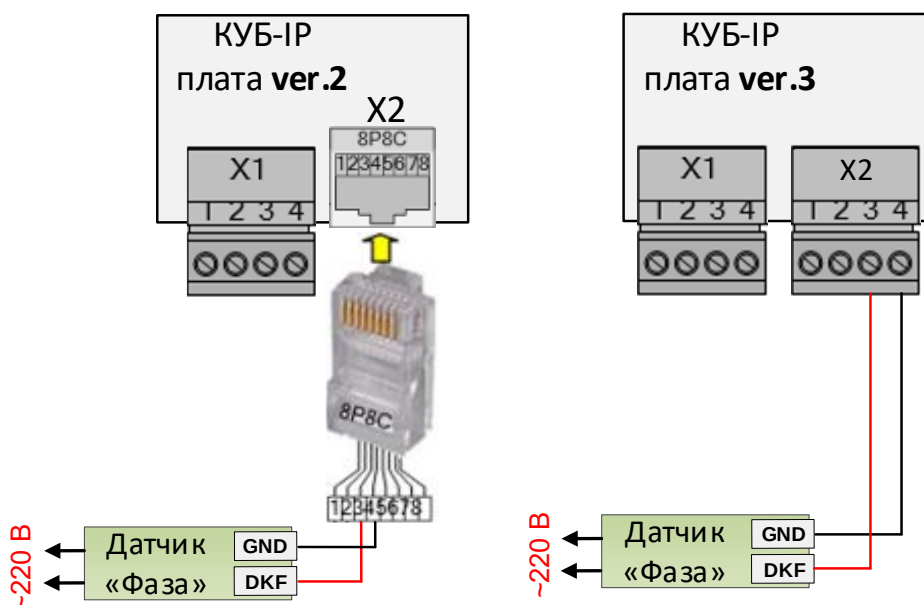
Рисунок 6. Подключение датчика фазы.
