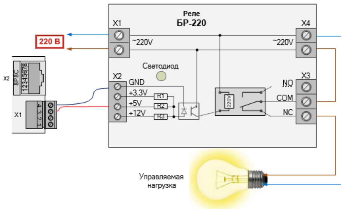
Рисунок 10. Подключение управляемой нагрузки с помощью внешнего реле
