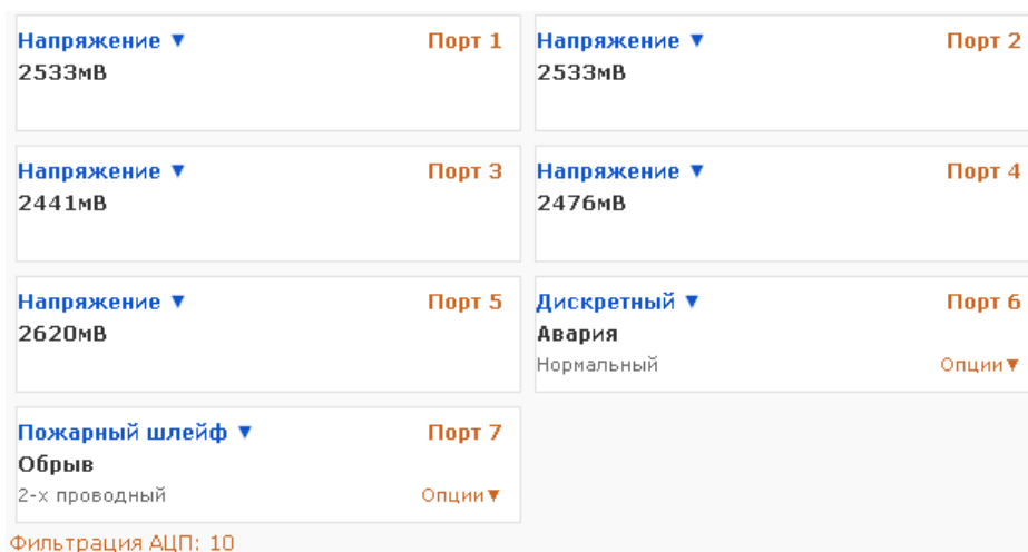
Рис.21. Конфигурация порта в качестве входа измерения напряжения
