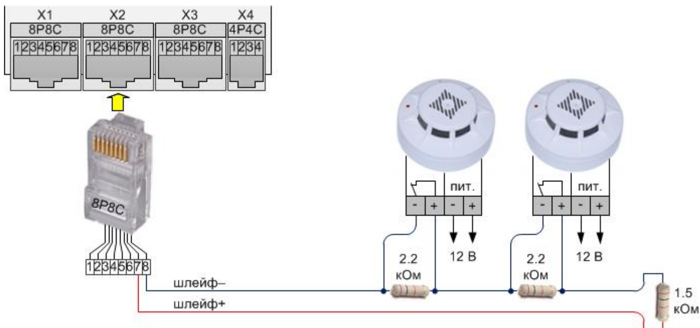
Рис.31. Подключение 4-проводных НЗ пожарных датчиков
