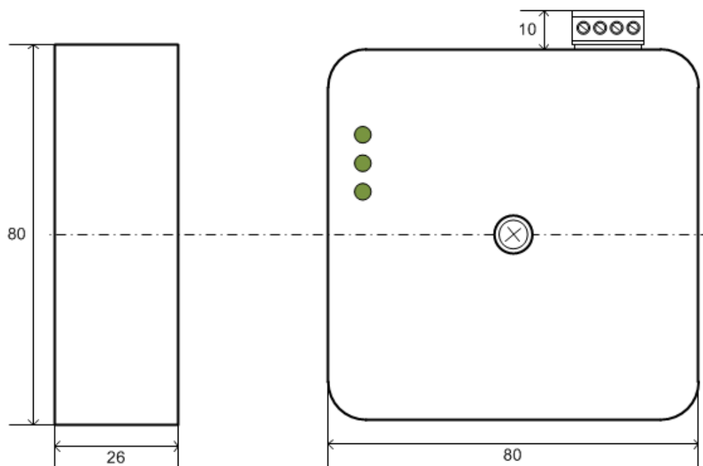
Рис.73. Габаритные размеры корпуса (без адаптера ДИН-рейки).
