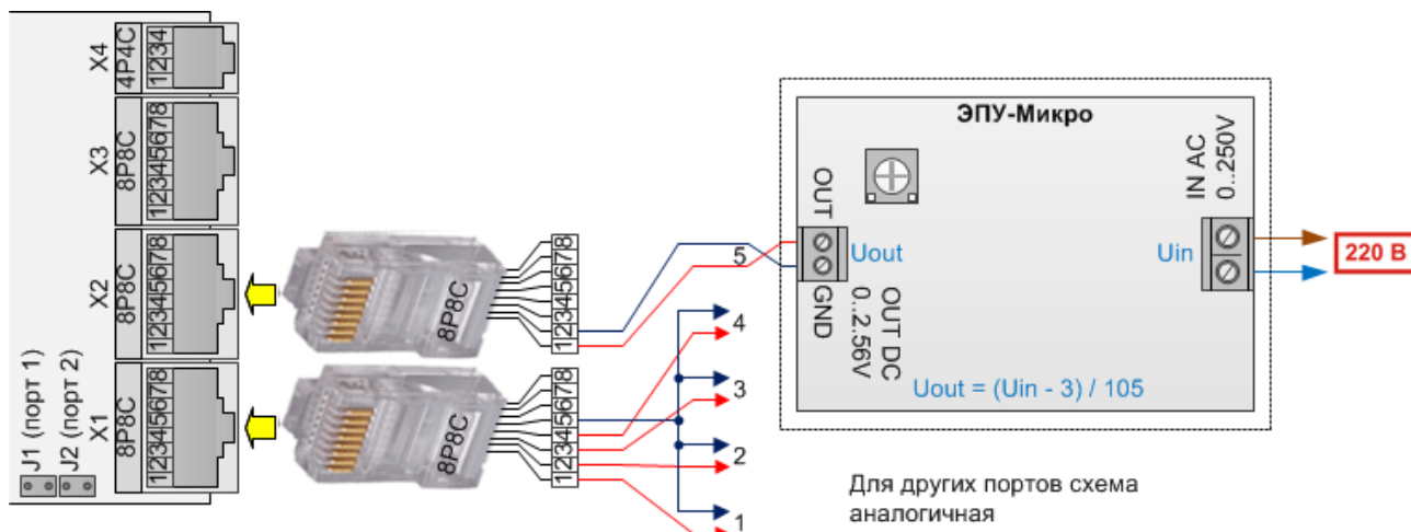
Рис.22. Подключение ЭПУ-Микро
